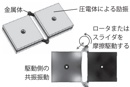
単相駆動型超音波モータの構造例
