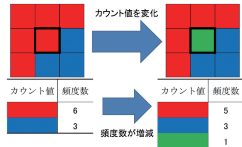
図1 電子透かしの埋め込み原理
