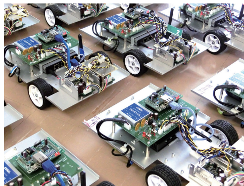
図1 インターネットから遠隔操作できるラジコン自動車
