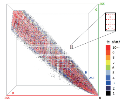
図2 3次元ヒストグラムへの電子透かしの埋め込み（「工大」が電子透かし）
