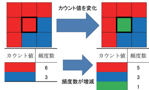
図1 電子透かしの埋め込み原理
