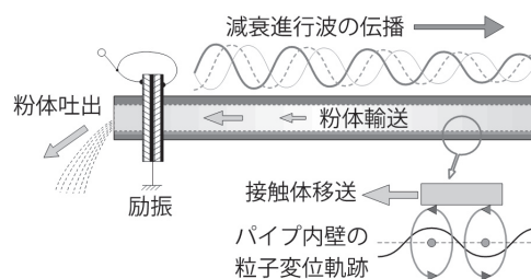
パイプ振動による粉体輸送の原理
