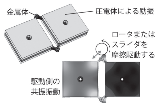
単相駆動型超音波モータの構造例
