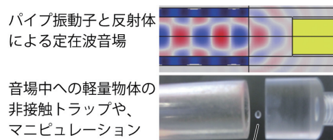
パイプ振動子による音場形成と非接触駆動
