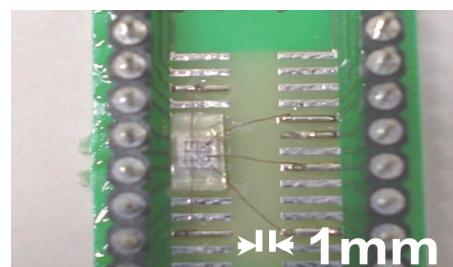
図3. 試作した臭化タリウム（TlBr）検出器
