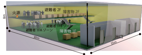
図2 建築図面（ケーススタディ）
